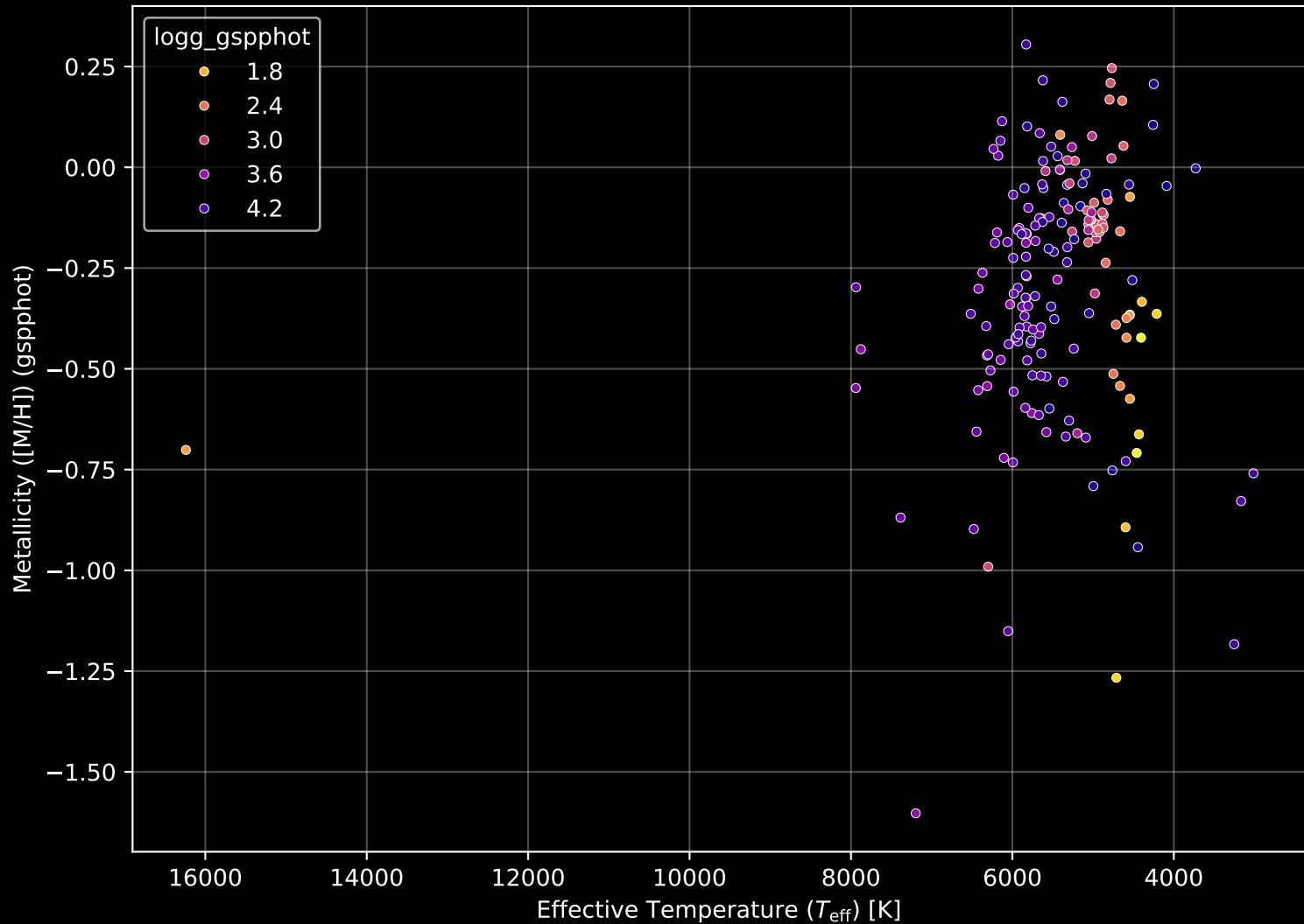
APOGEE DR17 Field: [284-26-O_TESS] Stellar Population Parameters (n= 180)
