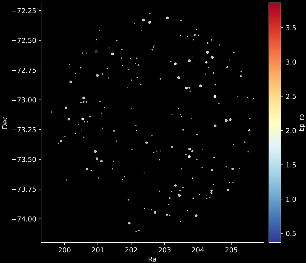
APOGEE DR17 Field: [284-26-O_TESS] Stars: 180
